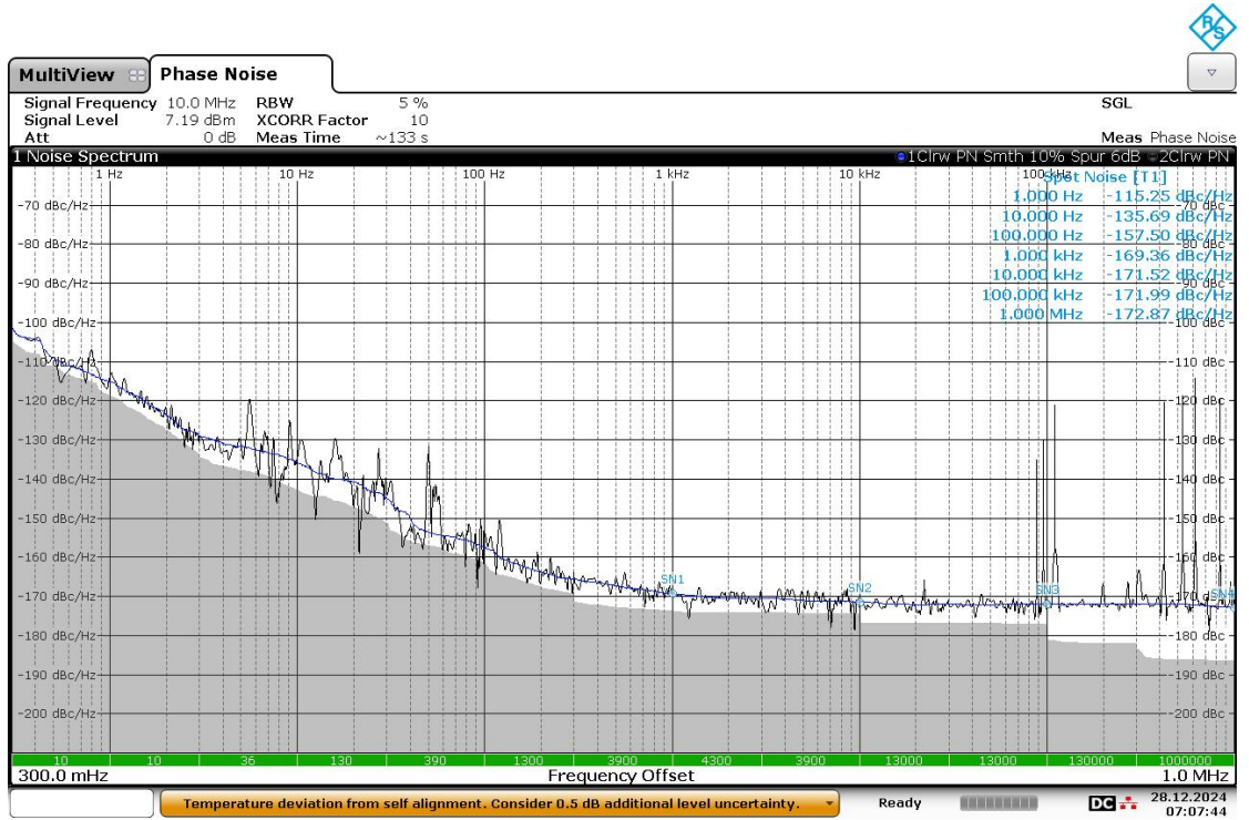
10MHz 相位噪声测试图
