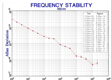
上图为主从节点频率附加稳定度测试数据
