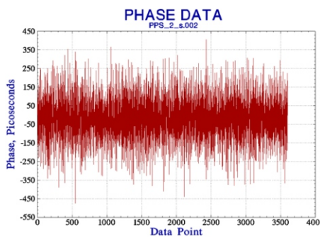
上图为主从节点时间同步测试数据
